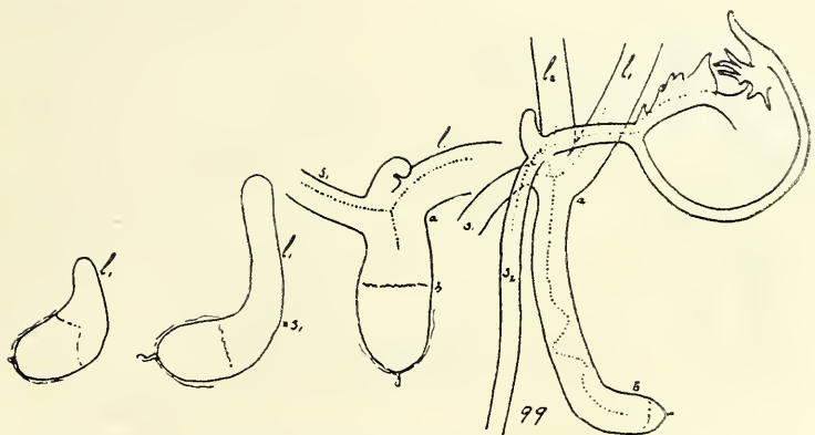
Fig. 6. Germination in U. monanthos .
